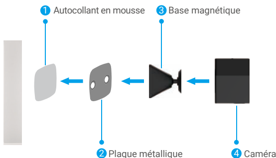
Fig.1 Montage à l'aide de l'autocollant en mousse
