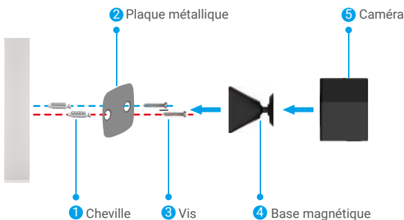
Fig.2 Montage à l'aide de vis
